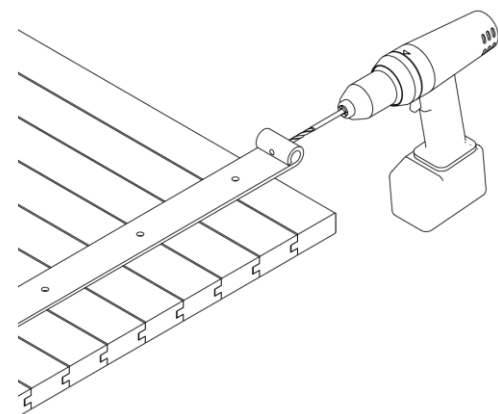
Perçage parallèle
