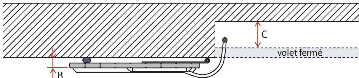
Abaque bras W2 & W3 pour une profondeur C ≥ 100 mm
